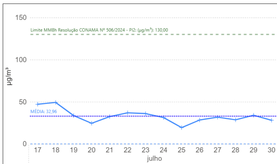
Figura 15 - Máximo da média móvel 8h para o ozônio
