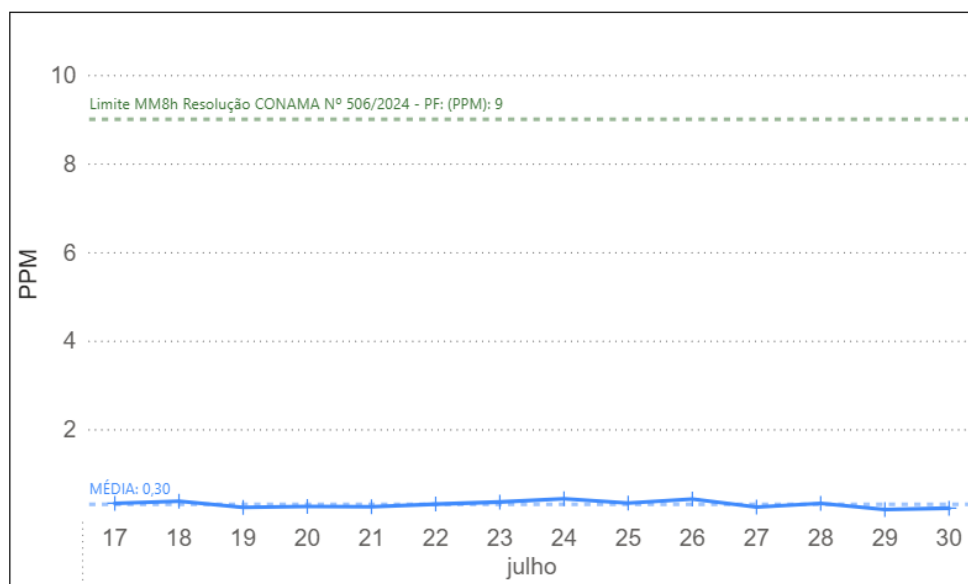
Figura 14 - Máximo da média móvel 8h CO
