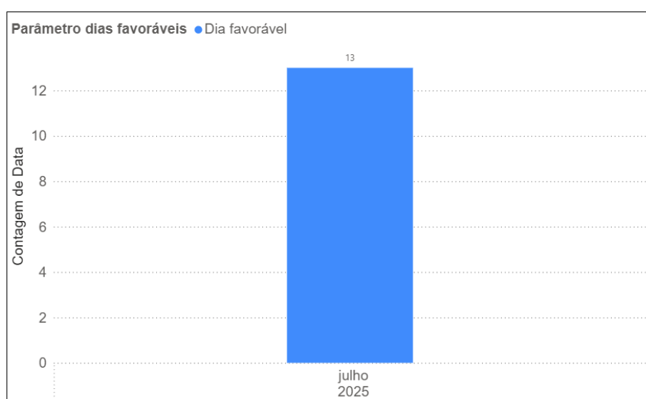
Figura 8 - Dias favoráveis à dispersão de poluentes
